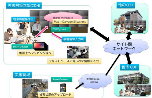
図 2. LIVEWall の概要
