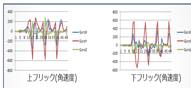
図7 角速度による上下フリックの判定
