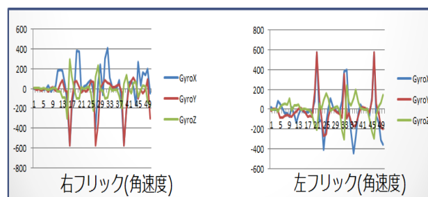
図8 角速度による左右フリックの判定
