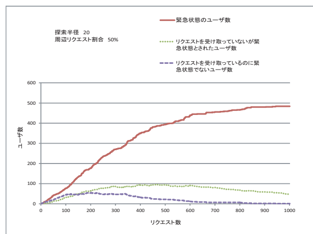
図 5 予備実験の結果
