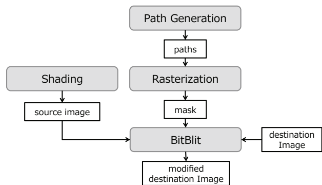
図1 Skia レンダリングパイプライン
