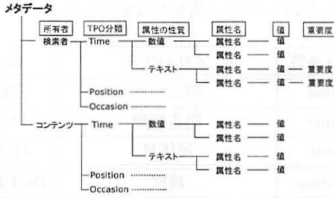
図 2: メタデータの分類
