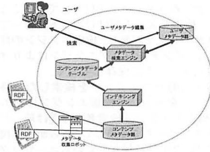
図 3: メタデータ検索エンジン
