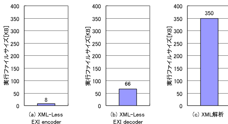
図 10 XML parser と XML-Less EXI の実行ファイルサイズ Fig. 10 Size of XML parser object file and XML-Less EXI object file.
