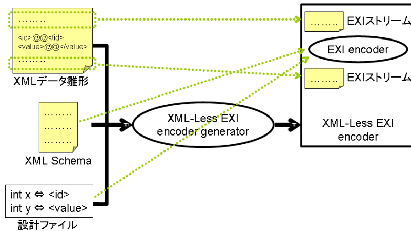
図 6 XML-Less EXI encoder generator の入出力 Fig. 6 XML-Less EXI encoder generator.
