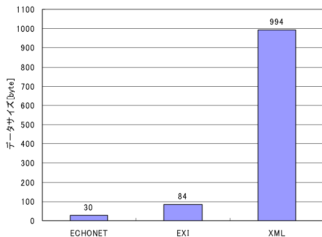
図 9 ECHONET と EXI と XML のメッセージサイズの比較 Fig. 9 Size of ECHONET message, EXI stream and XML document.
