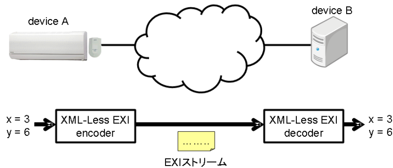
図 4 XML-Less EXI の利用例 Fig. 4 Example of XML-Less EXI-use case.
