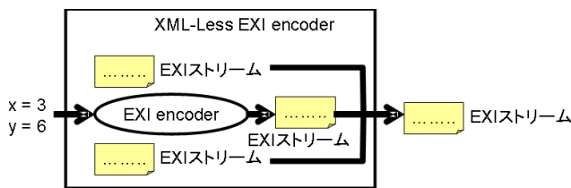
図 5 XML-Less EXI encoder の構成と動作 Fig. 5 XML-Less EXI encoder.
