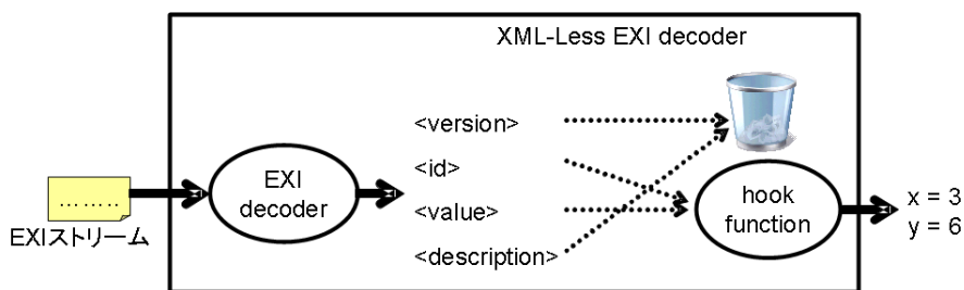
図 7 XML-Less EXI decoder の構成と動作 Fig. 7 XML-Less EXI decoder.
