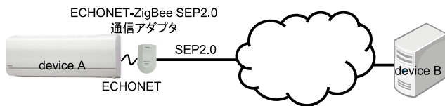
図 1 ECHONET-ZigBee SEP2.0 通信アダプタを含むホームネットワークの構成例
