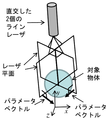
図 6 直交する 2 個のラインレーザによる形状計測.
