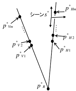
図 11 格子パターンが生成するパターン平面の双対空間中での配置. Fig. 11 Positions of the pattern planes generated by a grid pattern in dual space.
