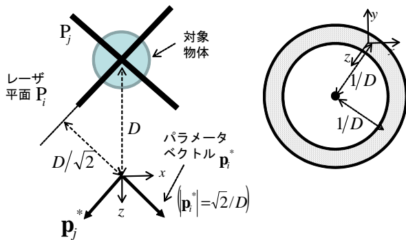
図 7 直交ラインレーザ投光器の典型位置 (左) と、レーザ平面の双対点の典型位置 (右)。
