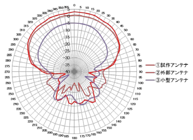
1980MHz帯における放射特性比較(金属板)
