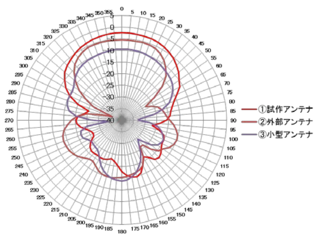
824MHz帯における放射特性比較(金属板)
