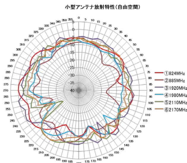
図 6 小型アンテナ放射特性 (自由空間)
