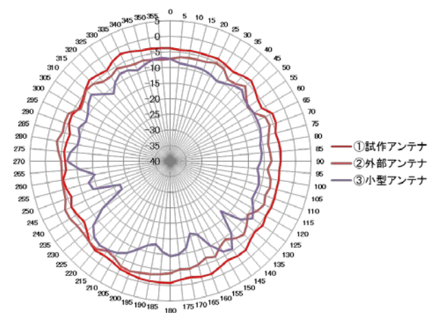
1980MHz帯における放射特性比較(自由空間)
