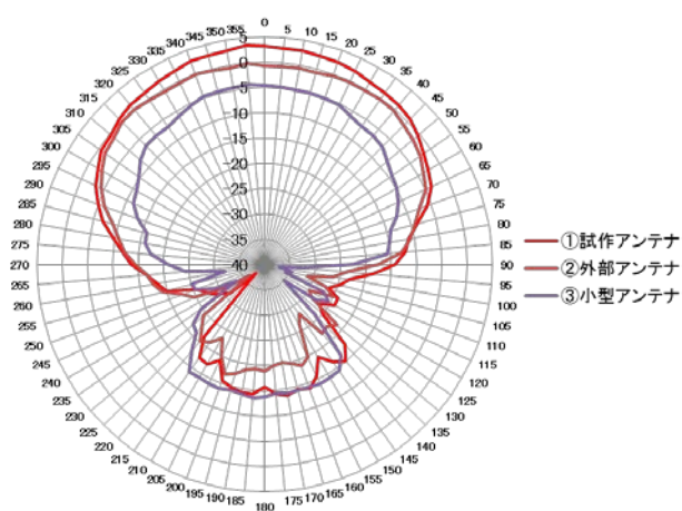
1920MHz帯における放射特性比較(金属板)
