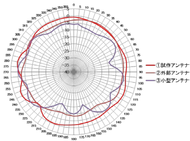
824MHz帯における放射特性比較(自由空間)
