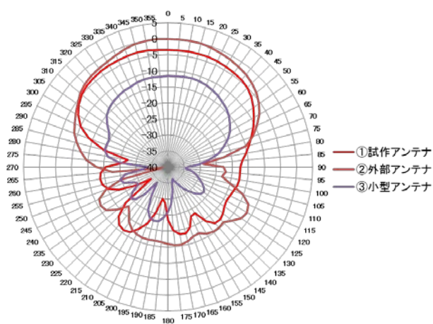
885MHz帯における放射特性比較(金属板)
