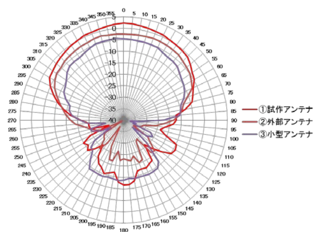
2170MHz帯における放射特性比較(金属板)
