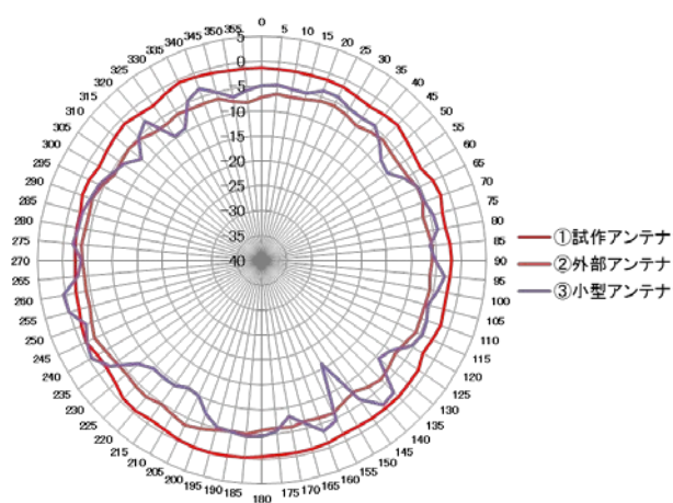
1920MHz帯における放射特性比較(自由空間)
