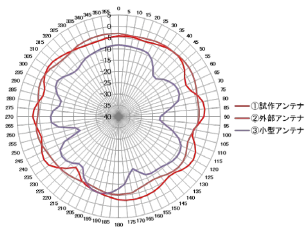
885MHz帯における放射特性比較(自由空間)
