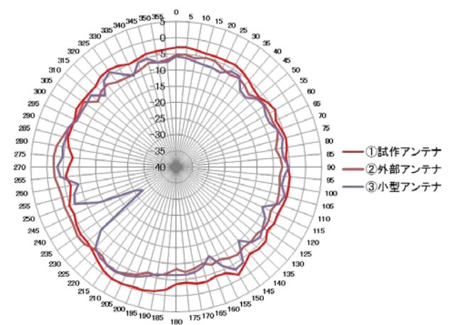
2110MHz帯における放射特性比較(自由空間)
