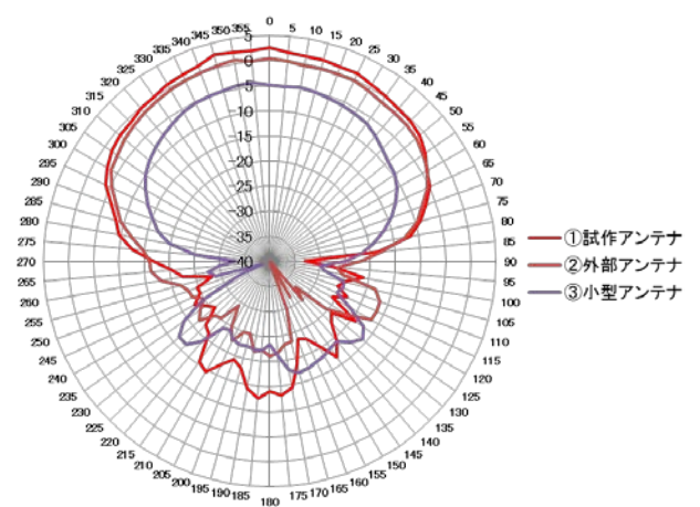
2110MHz帯における放射特性比較(金属板)
