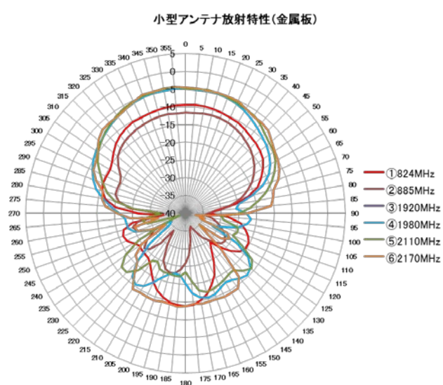
図 8 小型アンテナ放射特性 (金属板)
