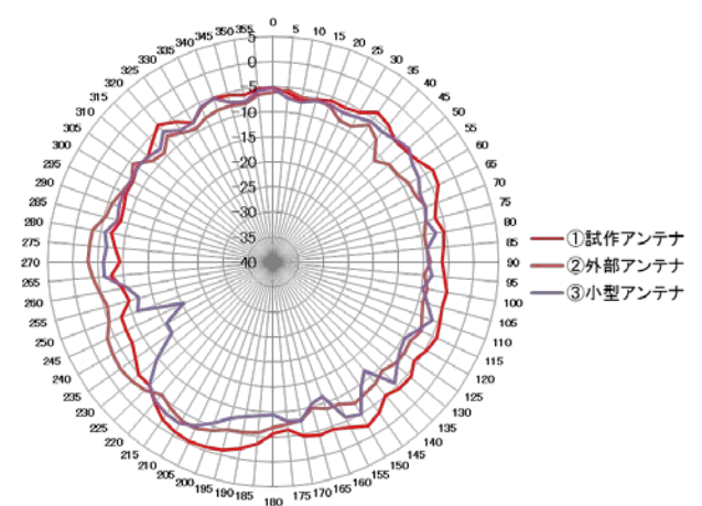
2170MHz帯における放射特性比較(自由空間)
