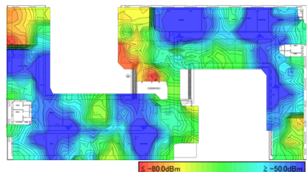
図 5 RSSI 測定値 Fig. 5 Measured RSSI
