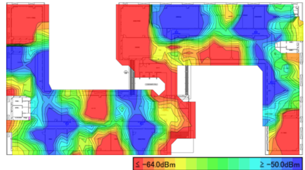
図 6 2.4GHz帯のRSSI
