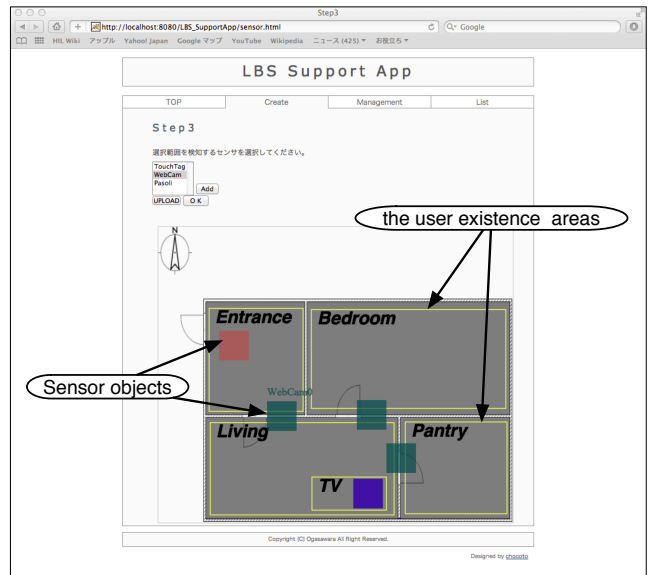
図 9 SASS 利用時のスクリーンショット Fig. 9 The screenshot of SASS
