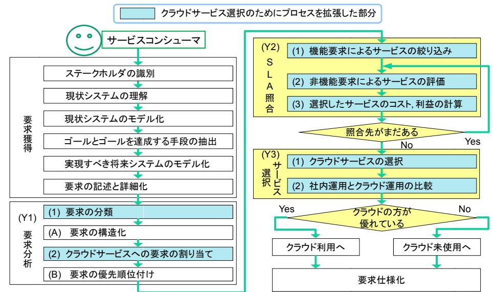
図2 提案するクラウドサービス選択プロセス
