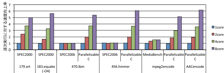
図 2 IBM p5 550Q における並列性能評価
