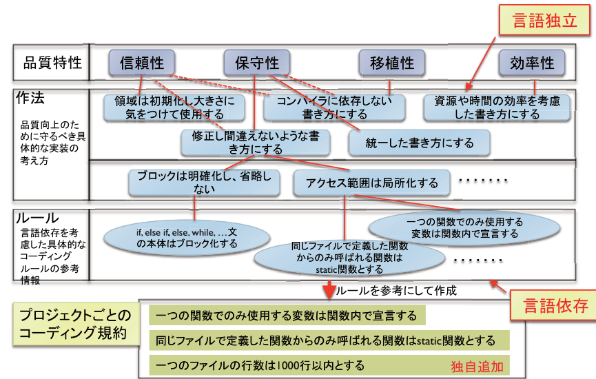
図1 品質特性、コーディング作法、コーディングルール、及びコーディング規約の関係
