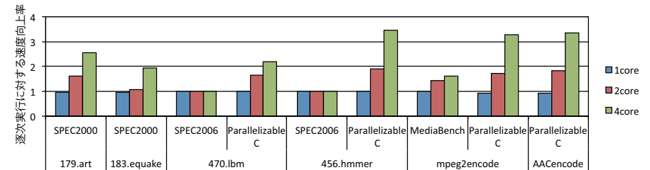
図 4 Renesas/Hitachi/Waseda RP2 における並列性能評価
