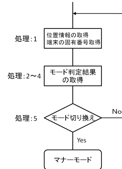
図 6 端末側の処理のフローチャート
