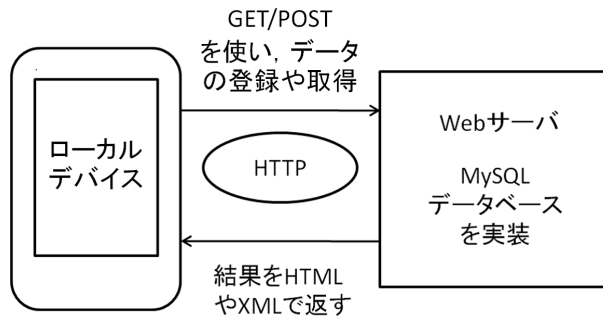
図 5 端末とサーバの通信の一例
