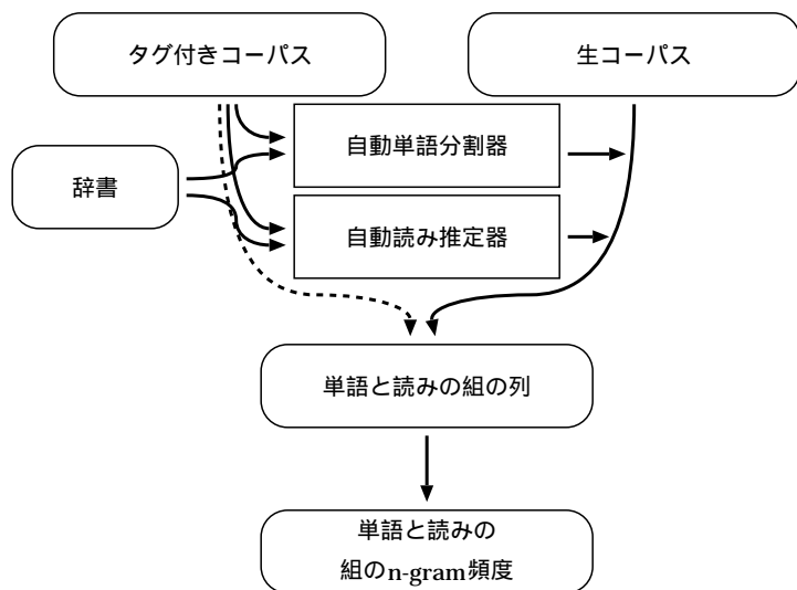
図 2 単語と読みの組を単位とする言語モデルの作成の手順
