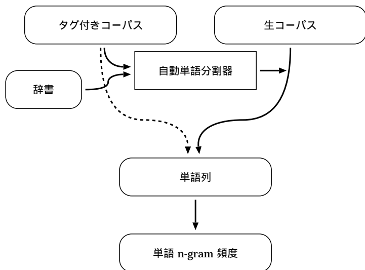
図 1 単語を単位とする言語モデルの作成の手順
