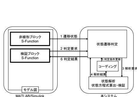
図 6 システム構成図 図 7 System Configuration
