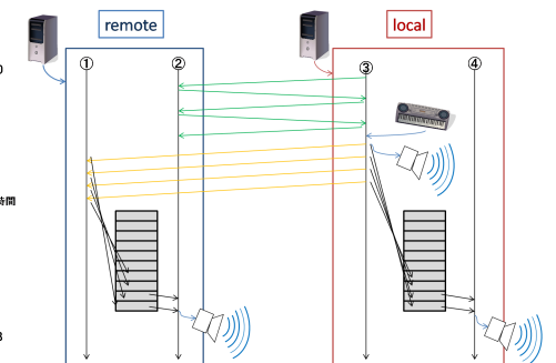
図 8 ローカル・ラグを実現するデータ・フローの概念 Fig. 8 Schematic diagram of data flow controlled by local lag.
