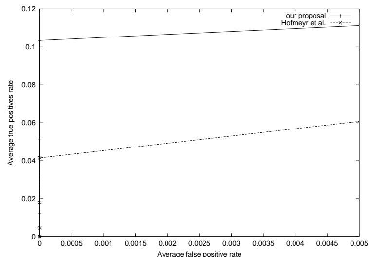
図6 psに関するデータを用いた異常検知の結果 (ROC 曲線) ( N = 6, D = 5 ) Fig. 6 The experimental result (ROC curve) using ps data set ( N = 6, D = 5 )
