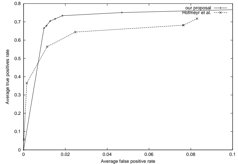
図 4 ftp に関するデータを用いた異常検知の結果 (ROC 曲線) ( N = 6, D = 5 ) Fig. 4 The experimental result (ROC curve) using ftp data set ( N = 6, D = 5 )
