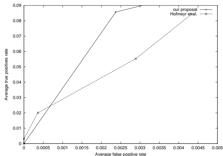
図5 loginに関するデータを用いた異常検知の結果 (ROC 曲線) ( N = 6, D = 5 ) Fig. 5 The experimental result (ROC curve) using login data set ( N = 6, D = 5 )
