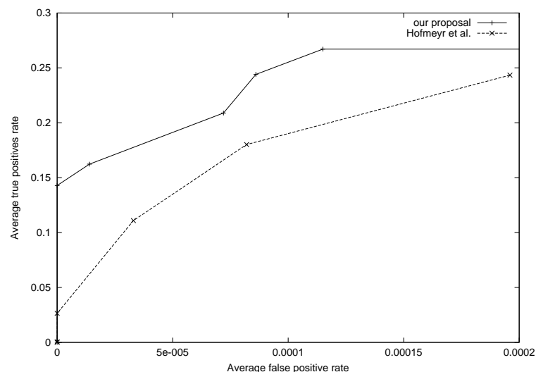
図 7 sendmail に関するデータを用いた異常検知の結果 (ROC 曲線) ( N = 6, D = 5 ) Fig. 7 The experimental result (ROC curve) using sendmail data set ( N = 6, D = 5 )
