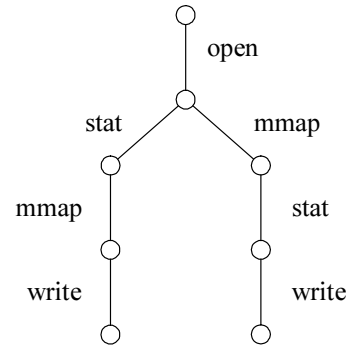
図2 sparse Markov tree の例 6) (4-gram の場合)
