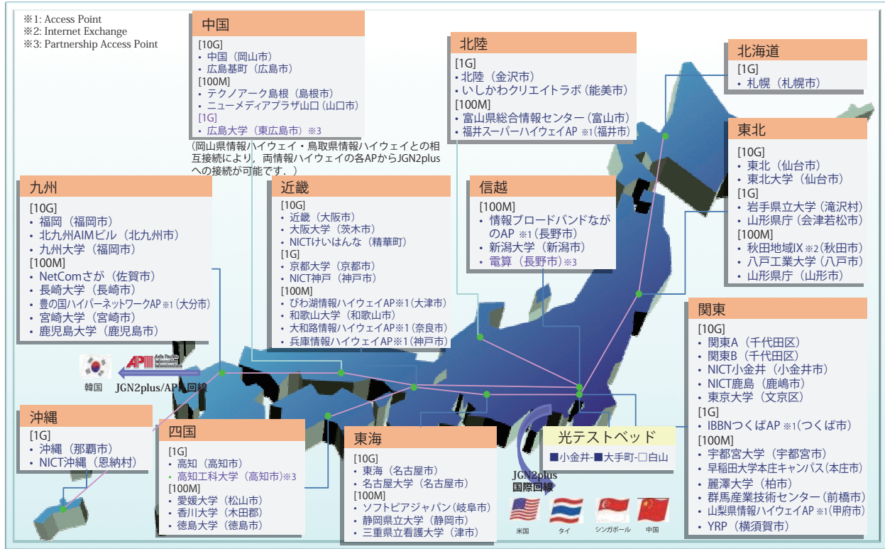
● 図-1 JGN2plus ネットワーク構成
