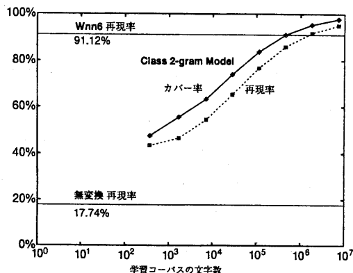
図 1: 学習コーパスの大きさと再現率の関係
