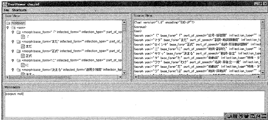
図 5: TreeView による表示
