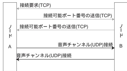
図 5: 音声通信経路の確立
