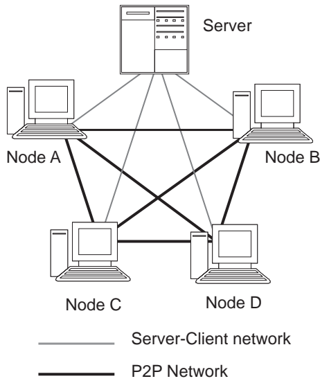
図 2: HybridP2P
