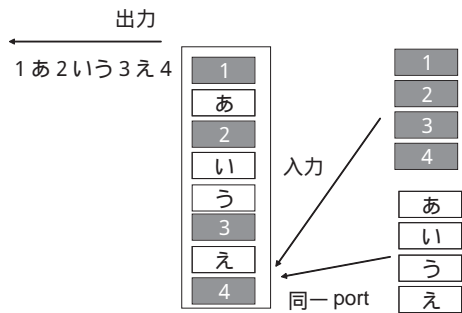
図 2: HybridP2P
