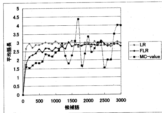
図 6: 各手法における 100 語毎の平均語長
