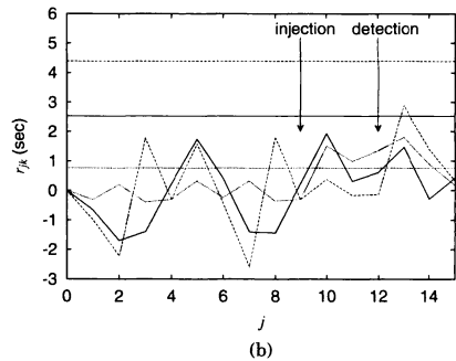
図4 監視開始後10分後にデータベースサーバーのバッファプールサイズを変化させることにより、性能問題を注入した際の、(a)各サーバーのサービスデマンドの推定値、(b)残差の時間変化を示す時系列グラフ。実線はウェブサーバー、破線はウェブアプリケーションサーバー、点線はデータベースサーバーの値を示す。
