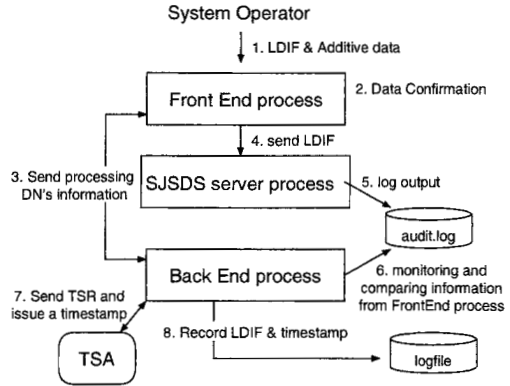
図 5: データ投入時のプログラムの振舞
