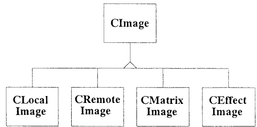
図 2: 映像クラスの派生関係
