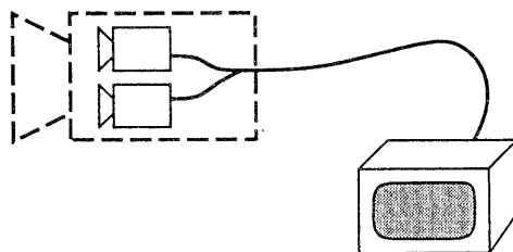
図 1: 仮想カメラ
