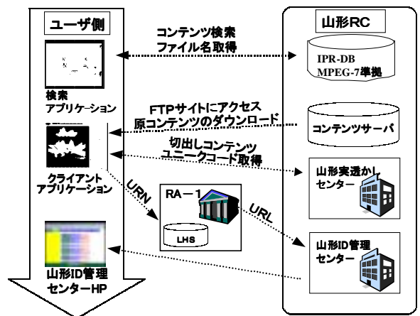
図 6 YRC 独自の検証実験 - 1 のフロー - 図 The original verification #1 tests flow of YRC
