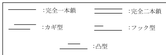
図 3 利用できる DNA 分子の形状 Fig. 3 Straightly formed molecular sequence figuration
