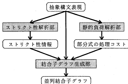
図5.1 並列結合子グラフ生成部の概要
