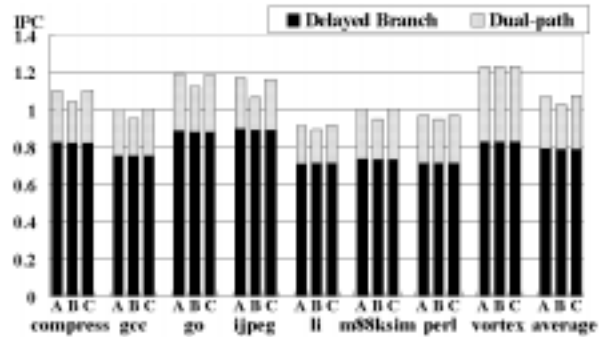
図 6: 各プロセッサの IPC (パイプライン段数 7 段)
