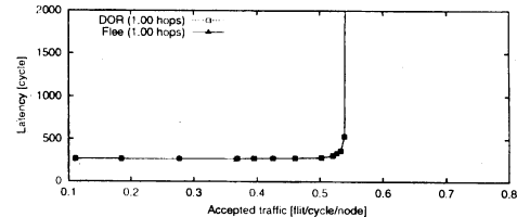
図 8 JPEG トレース (4 × 4 トラス)。
