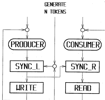
図5. 生産者消費者問題の実現
