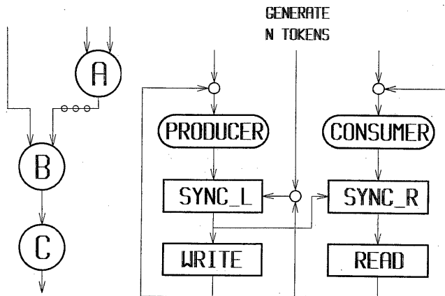
図5. 生産者消費者問題の実現
