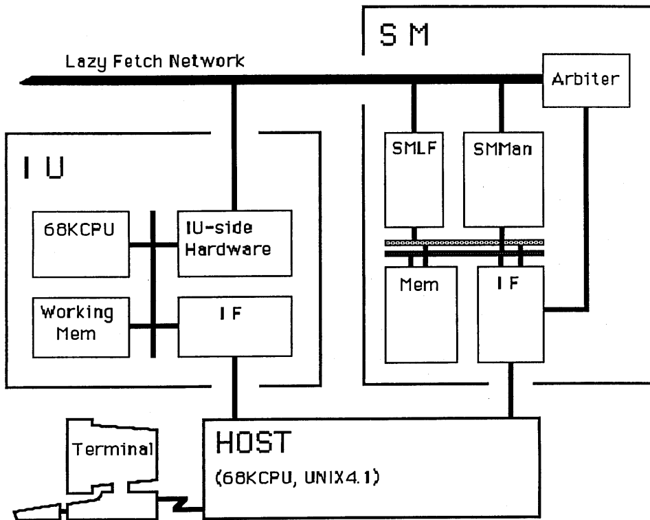
図1. 構造メモリ試作ハードウェアの全体構成
