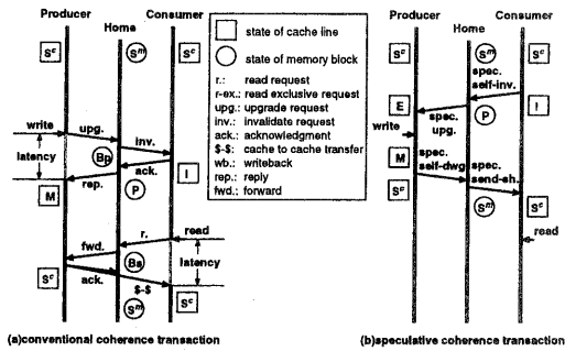
図4 PC共有状態における投機的コヒーレンス処理の例
