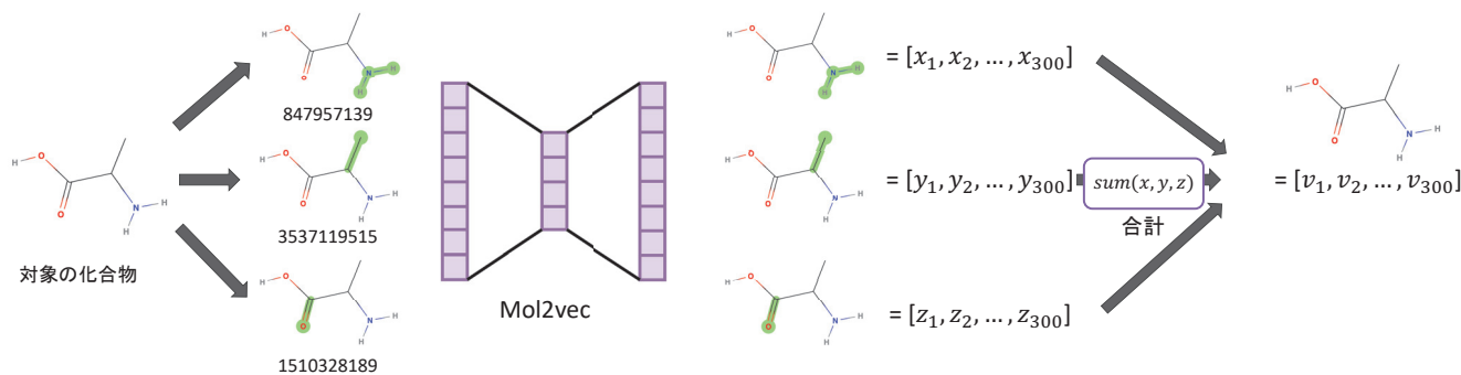
図 3: 化合物表現の構築
