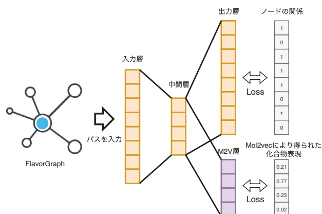
図 4: 食材表現の構築
