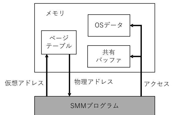
図 5 SMM プログラムにおけるアドレス交換
