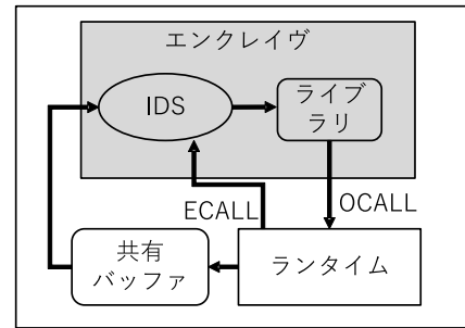
図 4 SGX アプリケーションの構成
