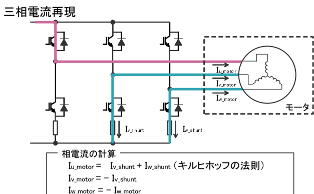
図 4 モータに流れる電流の仕組み
