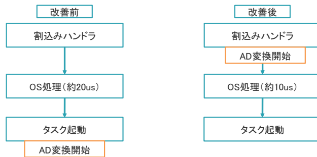
図 7 AD 変換タイミング変更の様子
