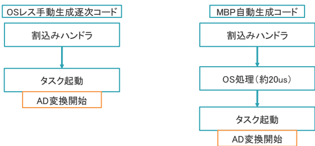
図 6 変更前の AD 変換タイミング
