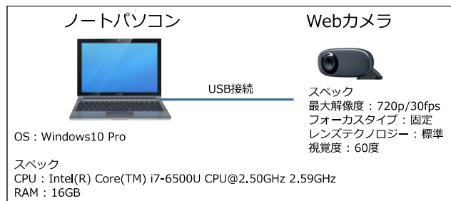
図 2 ハードウェア構成 Fig. 2 Hardware configuration.
