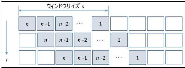
図 5 スライディングウィンドウ方式での時系列データ Fig. 5 Sliding window method for time series data.
