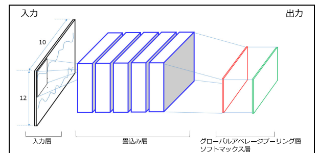
図 4 作業動作分類用のネットワーク Fig. 4 CNN for motion classification.
