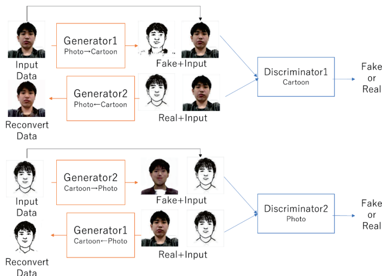
図 2 CycleGAN ペアの概要図. 顔画像から似顔絵を生成し, 顔画像に再変換を行う学習と似顔絵から顔画像を生成し, 似顔絵に再変換を行う学習がある. 生成した似顔絵から顔画像の生成を行う Generator2 を追加し, 再変換出来るようにしたネットワーク構造である. また, Generator2 を学習させる為に生成した顔画像と入力の似顔絵をペアにして Discriminator2 に識別させ, 結果を出力する.
