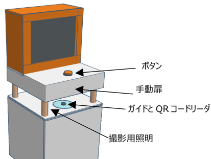
1-B コマスカウターの詳細 ディスプレイとボタン、撮影のためのUSBカメラと照明が設置されている。遮光のために全面に扉が設置されている。また内部にQRコードリーダが設置されているため、ガイドに独楽を置くことでQRコードを読み込める。
