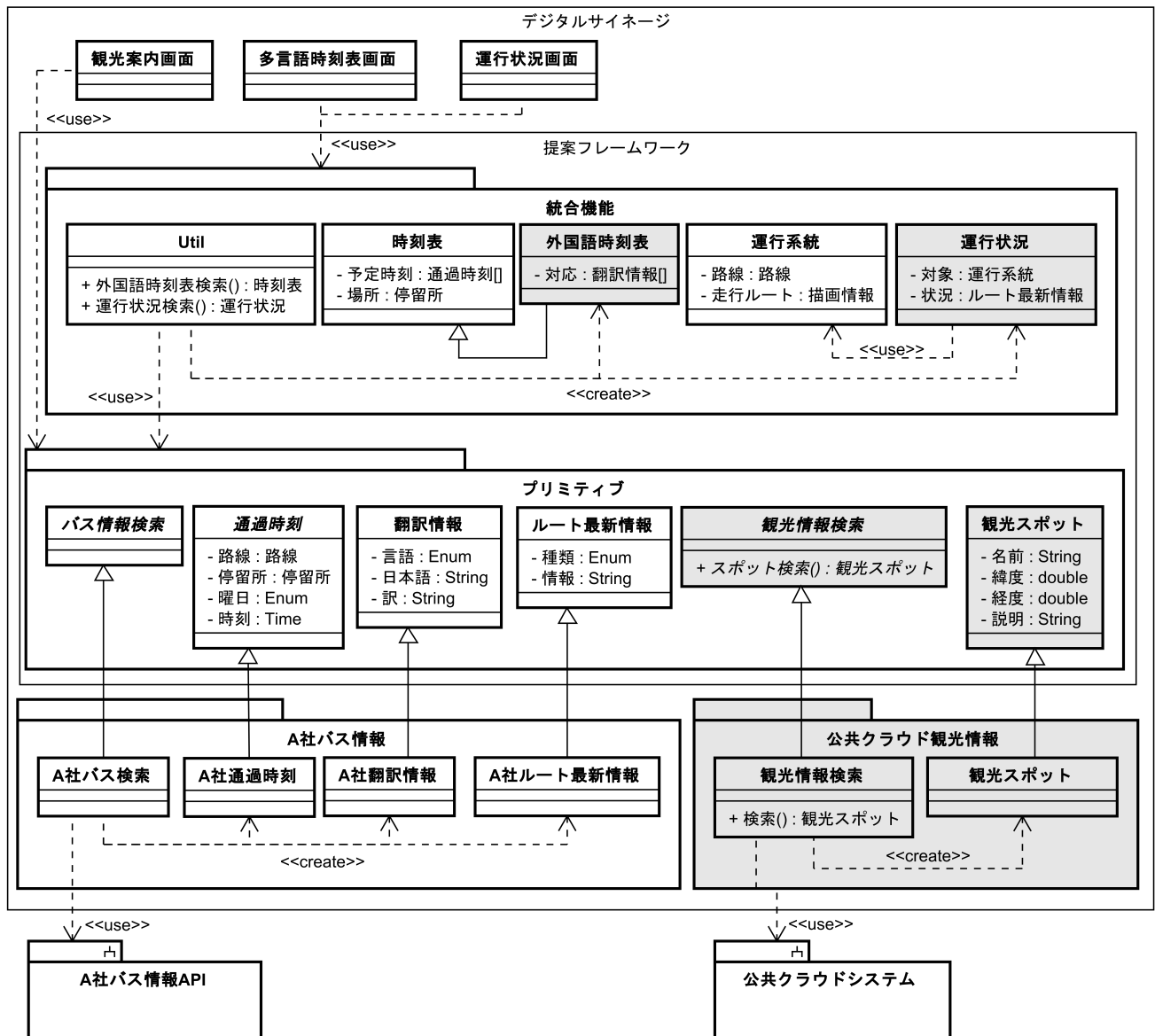
図 2 フレームワークを用いたデジタルサイネージのクラス図
