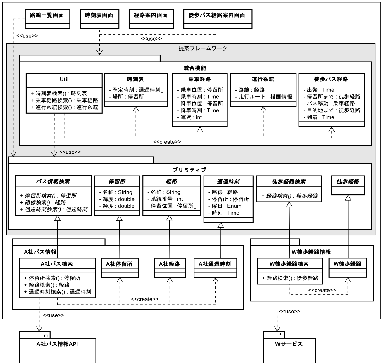
図 1 提案フレームワークを用いたシステムのクラス図
