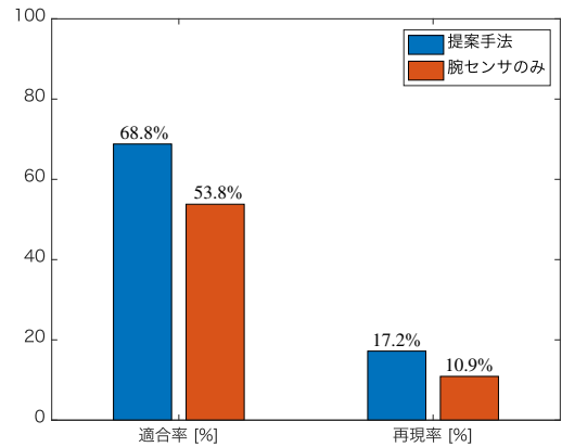
図 7 提案手法と腕センサのみによる手法の精度比較 エネルギー過剰消費状態=((温熱快適度)*HC > 0)
