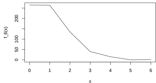
図 3 不動点数 f_6(x) の分布 ( k = 6 )
