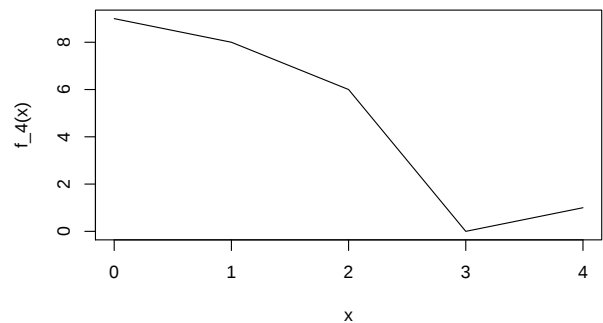
図 2 不動点数 f_4(x) の分布 ( k = 4 )
