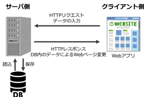
図 2 Stored XSS の概要
