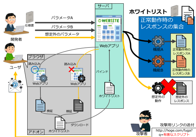
図 15 テストベースホワイトリストのデプロイ
