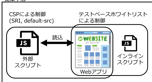
図 12 提案システムの概要図
