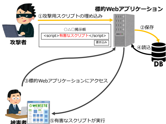
図 4 Stored XSS の仕組み
