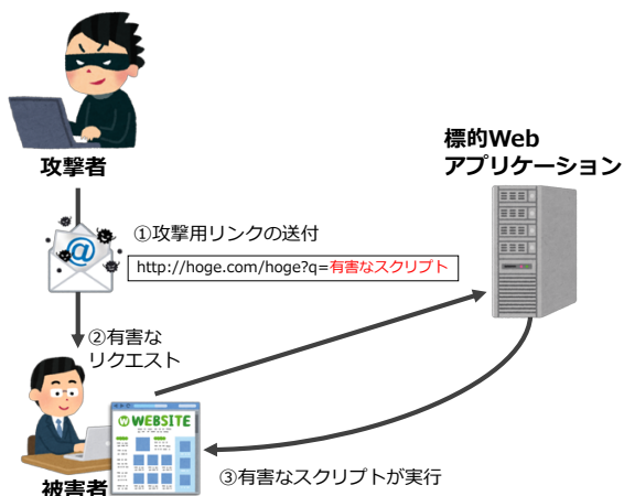
図 3 Reflected XSS の仕組み
