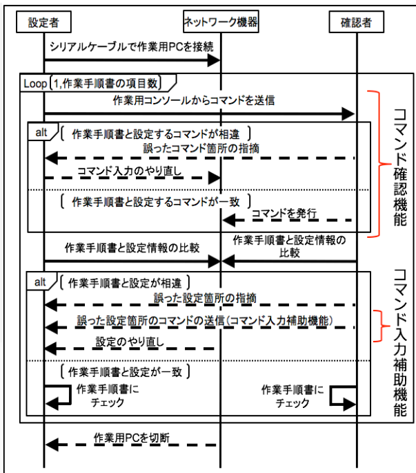
図 9 本システムを利用した ネットワーク機器管理のシーケンス図
