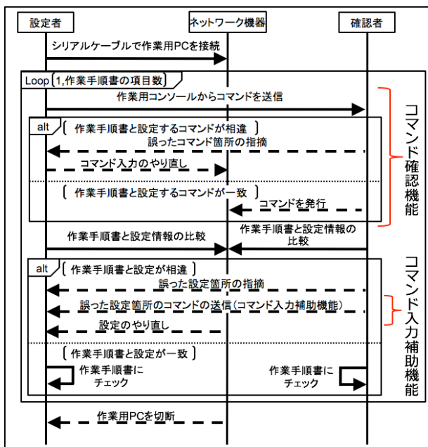
図1 現状のネットワーク機器管理のシーケンス図
