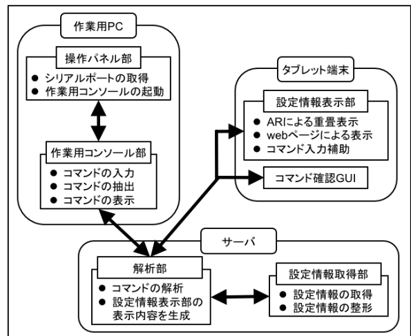
図 4 本システム構成
