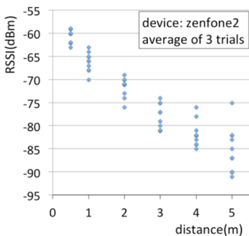
図 8. BLE 通信の距離と電波強度追加実験結果
