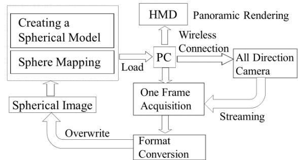
図 2 全天球映像呈示の流れ
