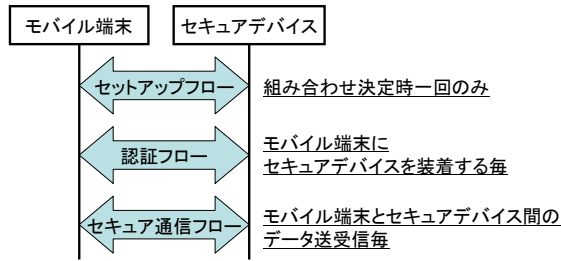
図2 処理フロー
