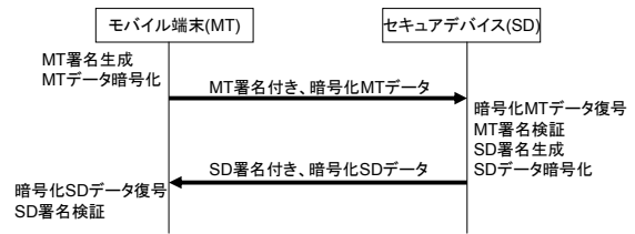
図5 セキュア通信フロー
