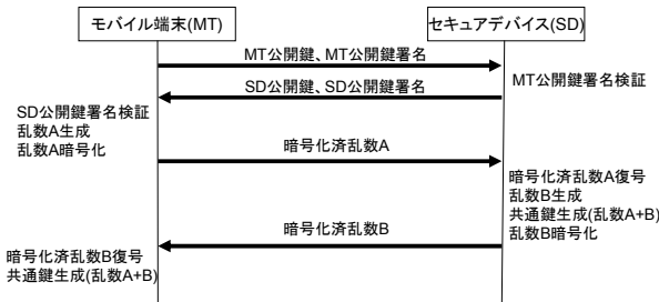
図3 セットアップフロー
