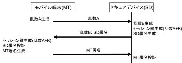
図4 認証フロー
