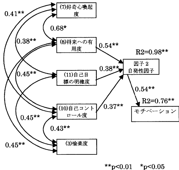
図2 中期 SIEM 構造分析パス図(2005年)
