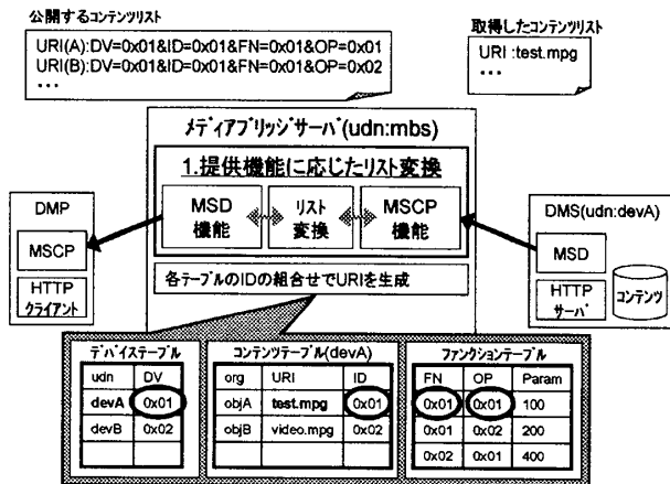
図3 コンテンツリスト生成処理 (URI の場合)
