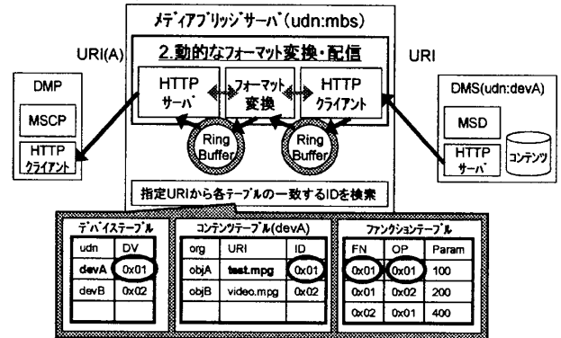
図4 動的なフォーマット変換処理
