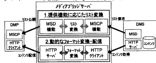
図2 メディアブリッジサーバの構成
