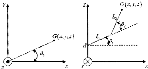
図1：逆運動学の数值的解法
